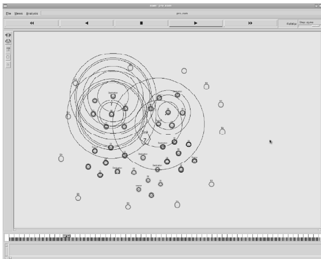
Figure 4: EM Maximization
