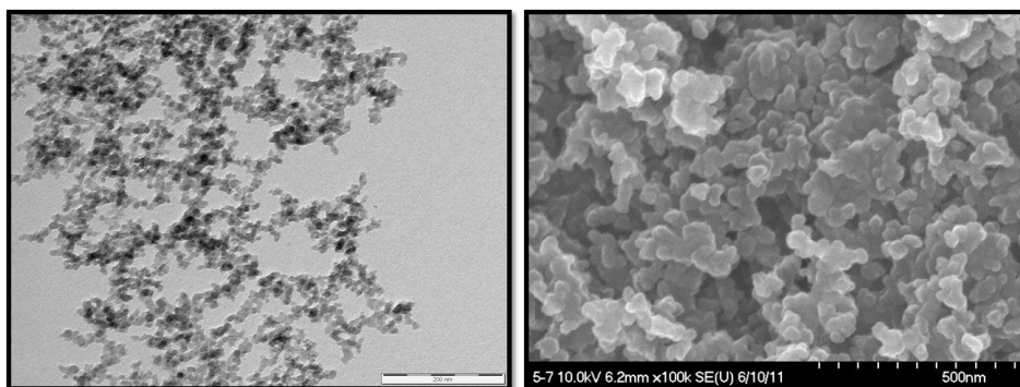
Figure 2: TEM & SEM images for the pyro Si, M-5.
